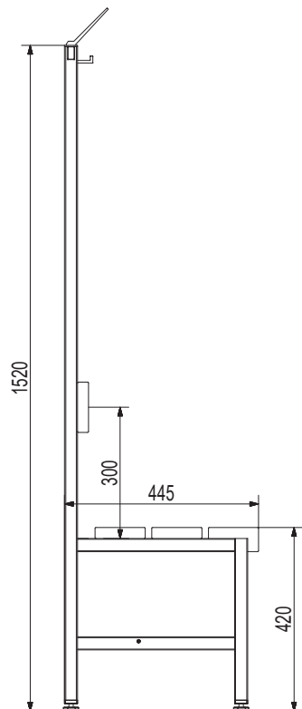
Bemassung Primarschule
