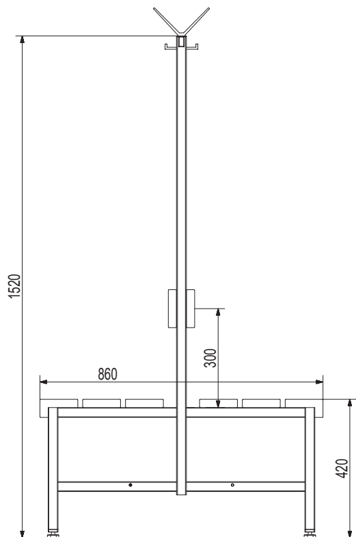
Bemassung Primarschule
